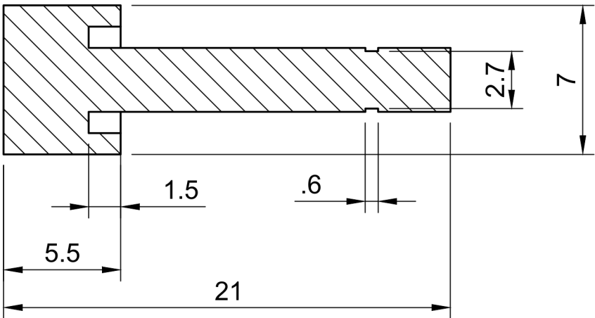
A-A (4:1)
